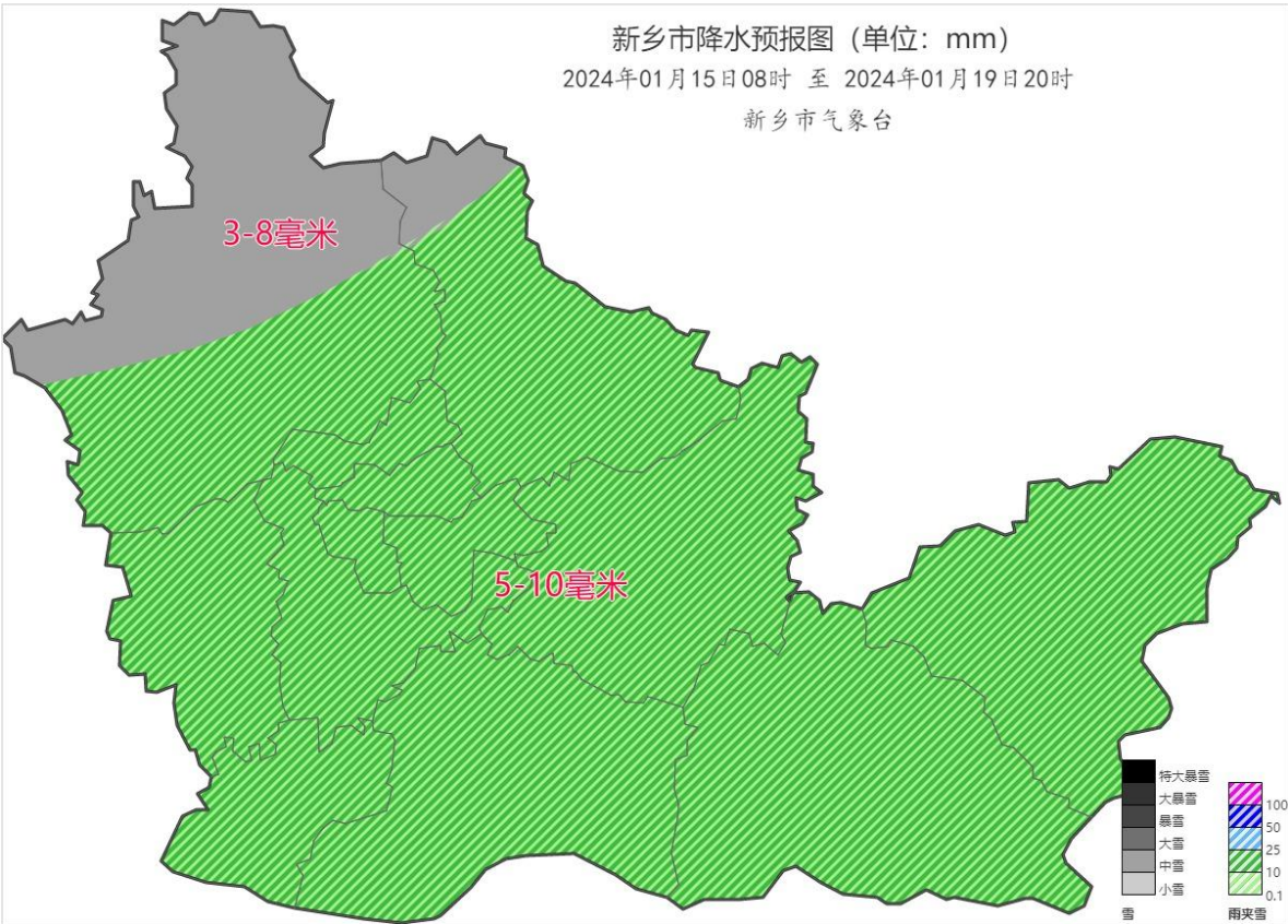
图 1: 2024 年 1 月 15 日 08 时至 19 日 20 时新乡市降水量预报图
